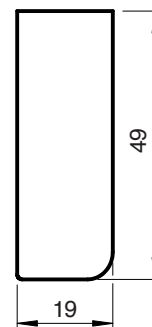
Lichtleiste
